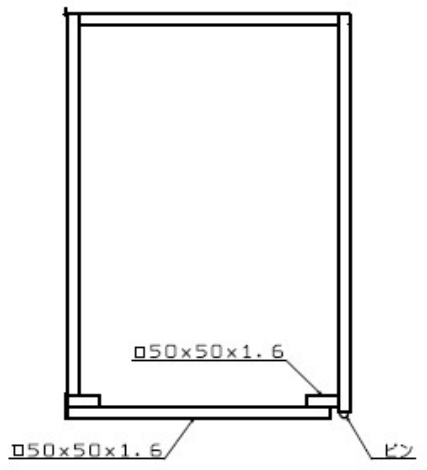
左側面図
