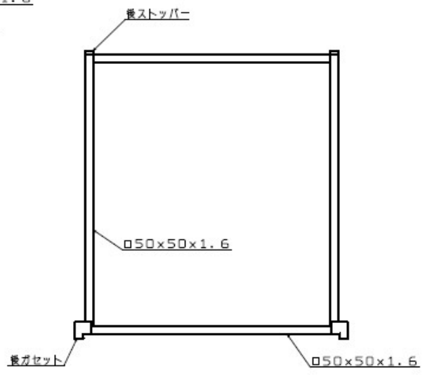
背面図
